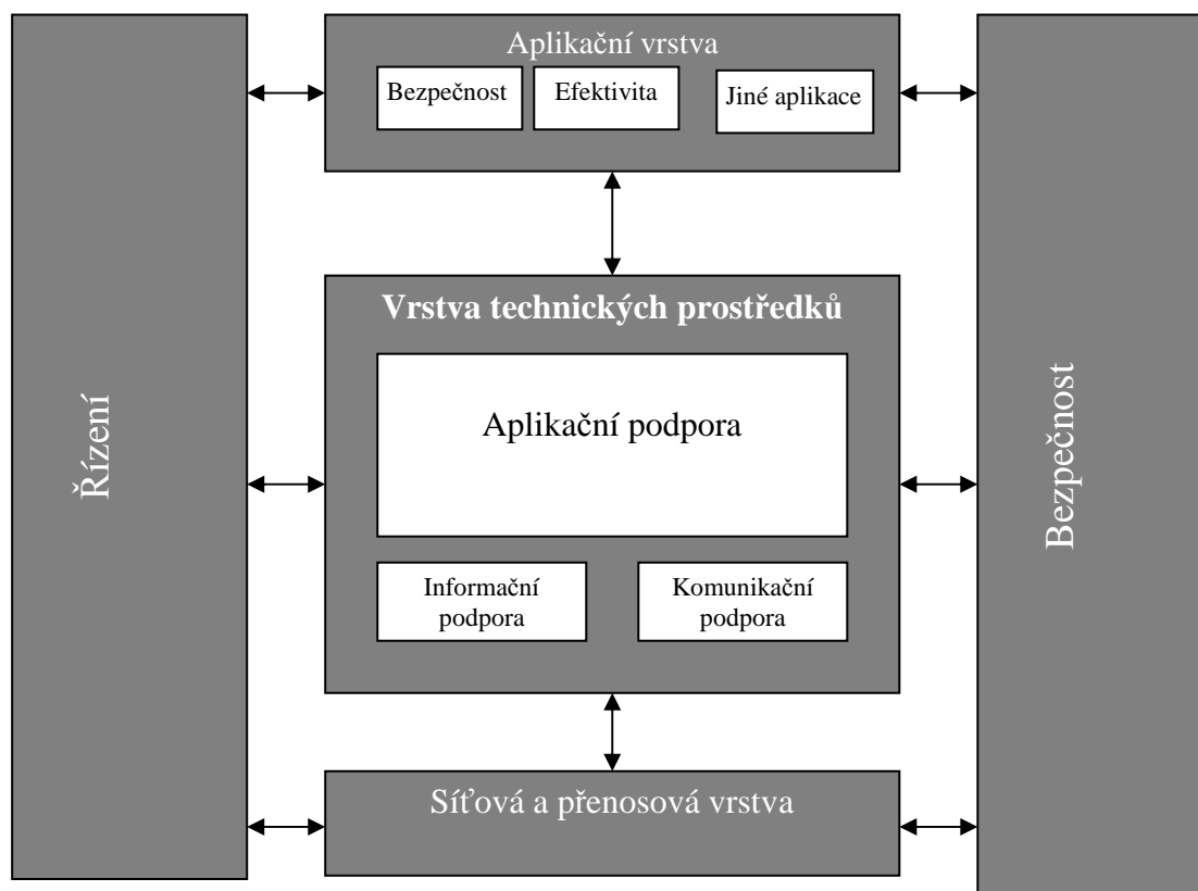
Obr. 1 – Referenční architektura stanic kooperativních systémů (OBU, RSU)
