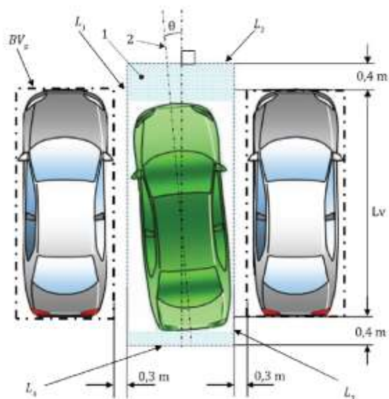
Obrázek 5 – Definice cílové oblasti a úhlu natočení vozidla pro případ kolmého parkování (obr. 15 normy)
