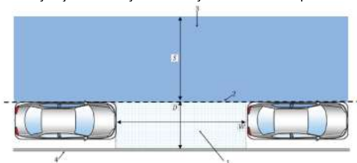
Obrázek 1 – Geometrie podélného parkovacího místa (obr. 1 normy)
