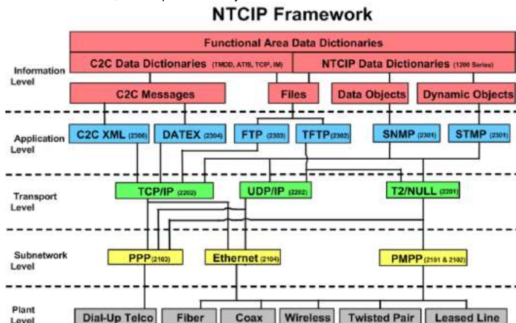
Obrázek 2 – Rámec NTCIP (obr. A.1 normy)
