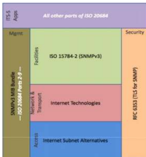
Obrázek 1 – Typický zásobník komunikace (obr. 1 normy)
