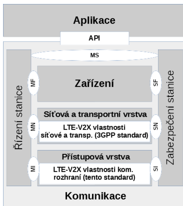
Obrázek 3 - LTE-V2X funkcionální v rámci stanice ITS (obr. 3 normy)
