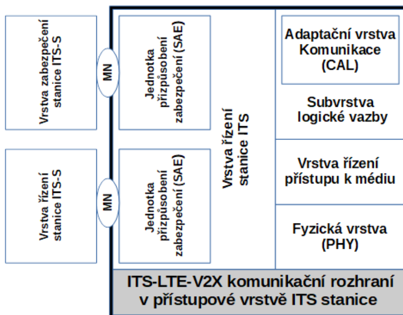
Obrázek 2 - Architektura komunikačního rozhraní LTE-V2X (obr. 2 normy)
