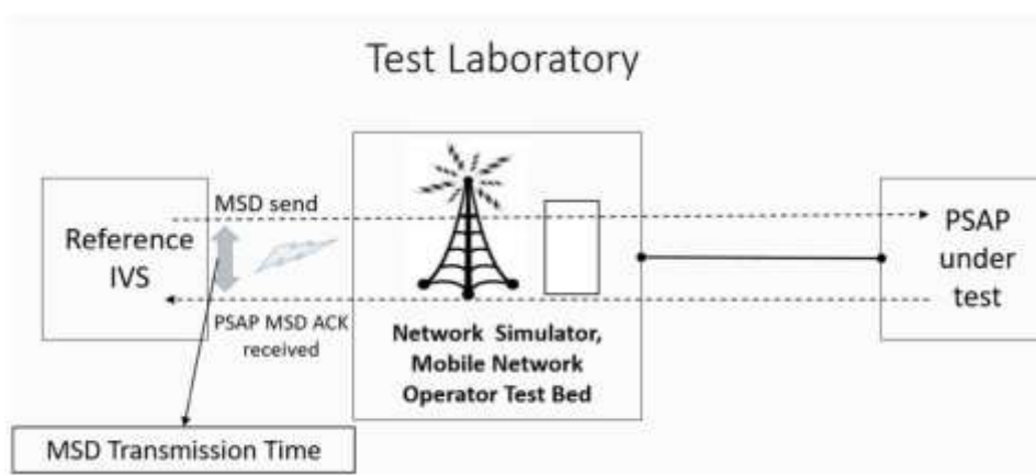
Obrázek 1 – Uspořádání testovací laboratoře (Obr. 4 normy)
