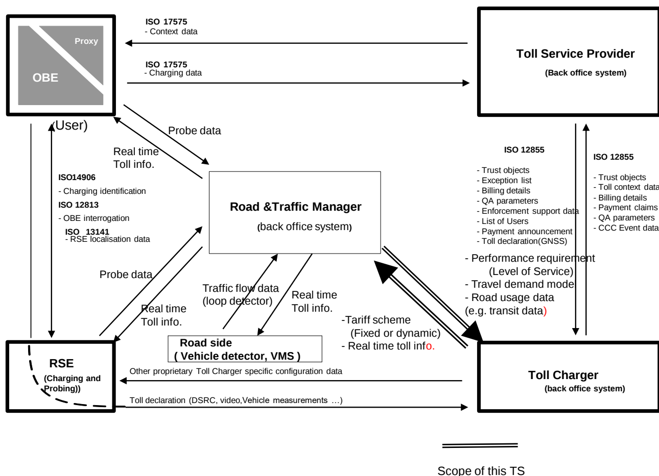
Obrázek 3 – Model datových toků mezi EFC systémem a správcem silnic a řízením dopravy (obr. H.1 normy)
