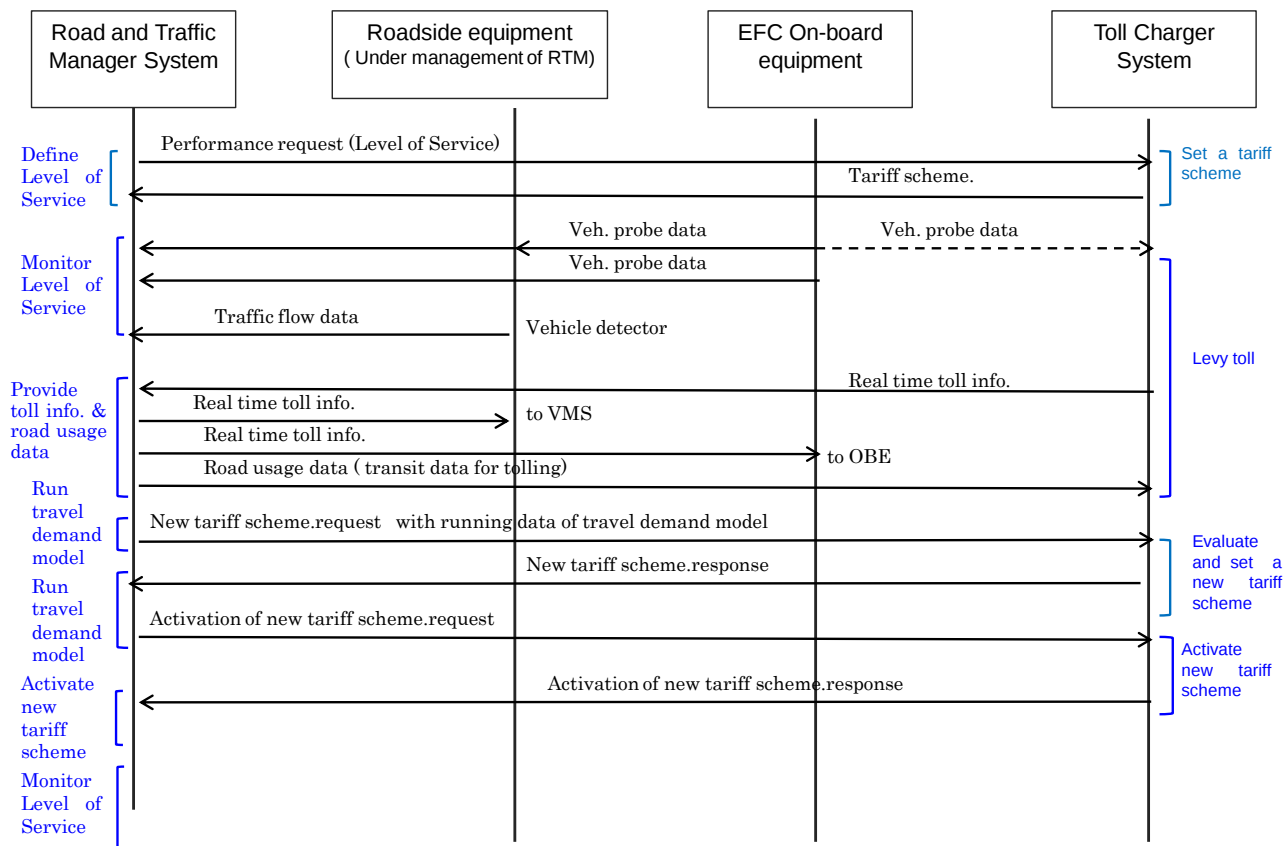
Obrázek 4 – Datové toky (obr. I.1 normy)
