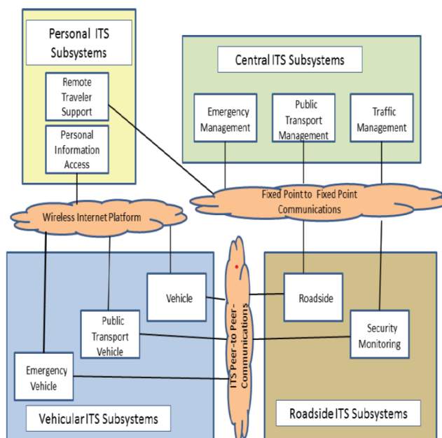
Obrázek 4 – Subsystém ITS v interakci s PT-DSS EEDRR (obr. 2 normy)
