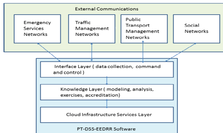
Obrázek 5 - Centralizovaná architektura PT-DSS EEDRR (obr. 3 normy)
