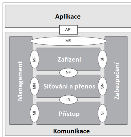
Obrázek 1 – Referenční architektura ITS-S stanice (obr. 1 normy)
