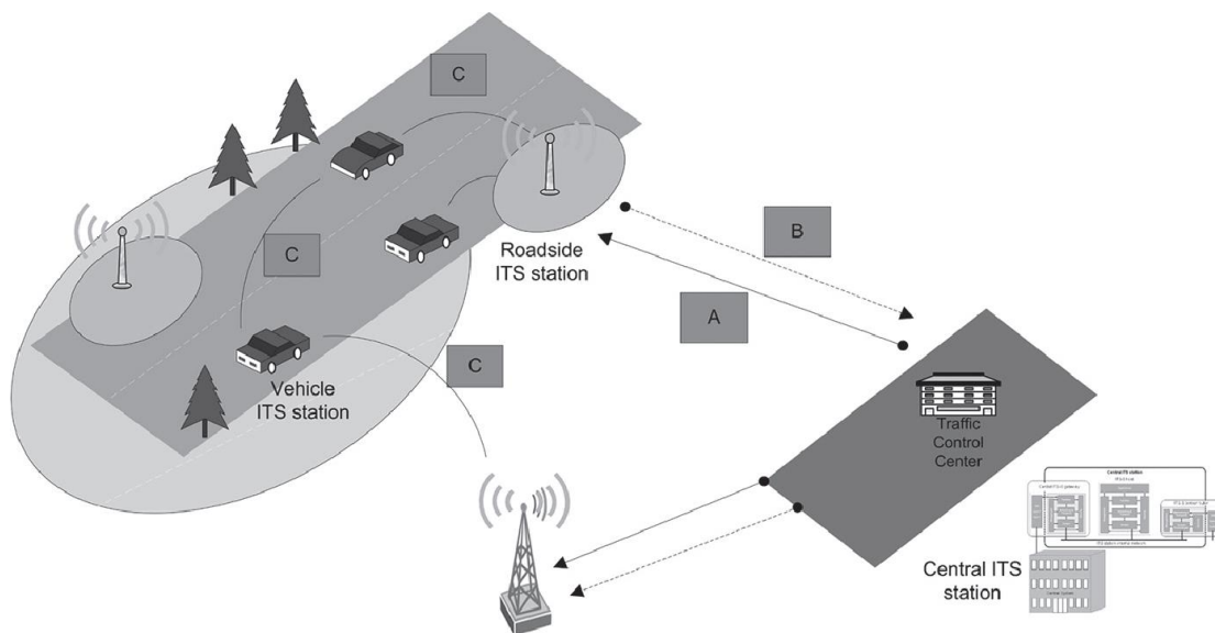
Obrázek 3 – Příklad architektury systému (obr. 7 normy)
