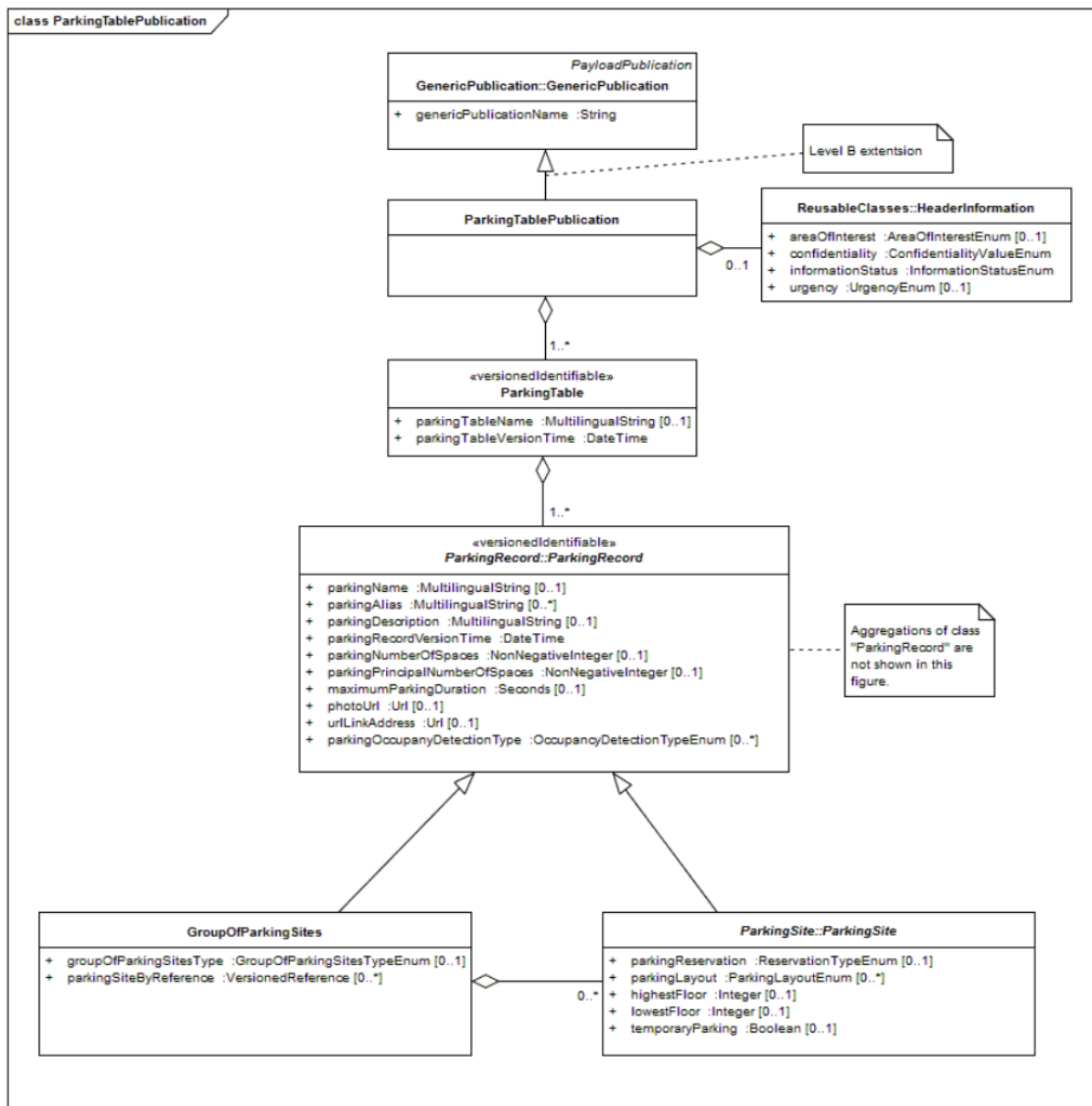
Obr. 1 - Model tříd balíčku "ParkingTablePublication": (obr. 2 normy)
