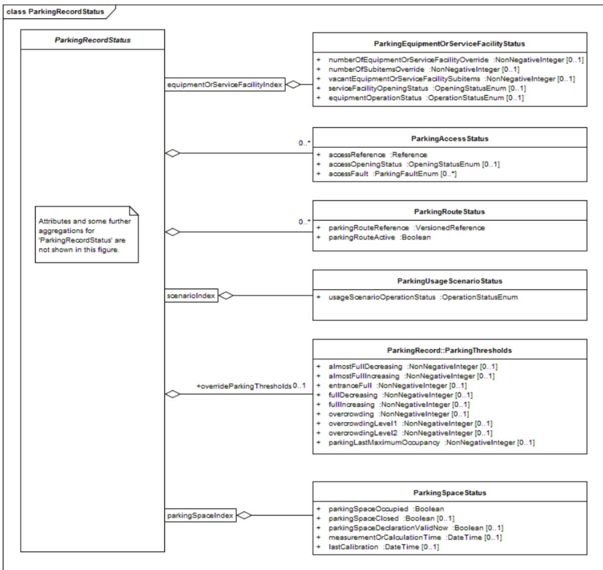
Obrázek 2 – Model tříd balíčku "ParkingRecordStatus"_(obr. 21 normy)
