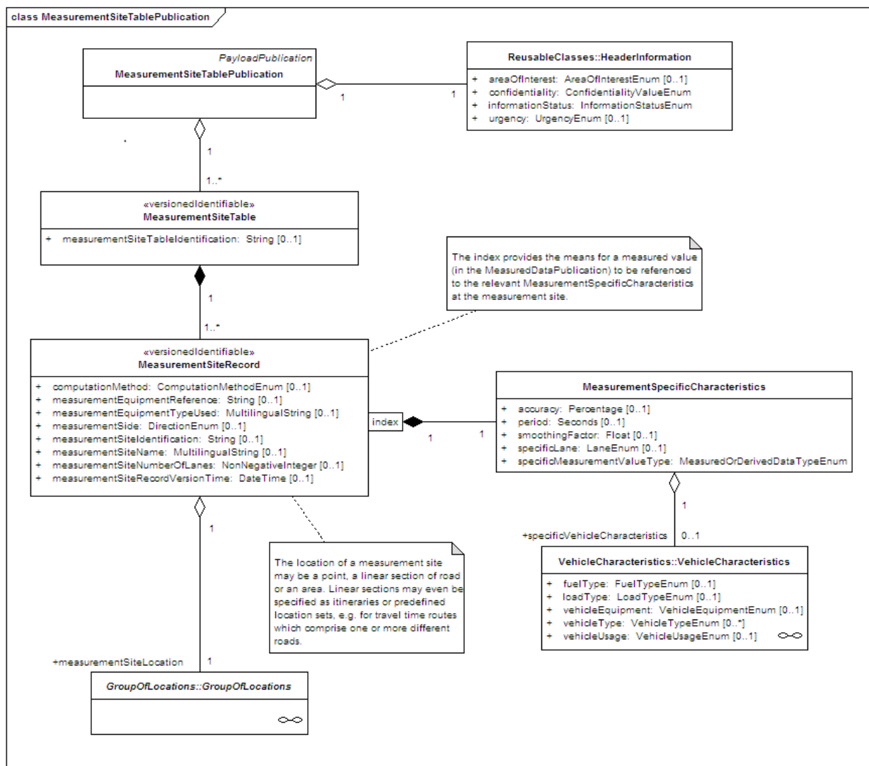
Obrázek 1 – Model tříd balíčku „MeasurementSiteTablePublication”
