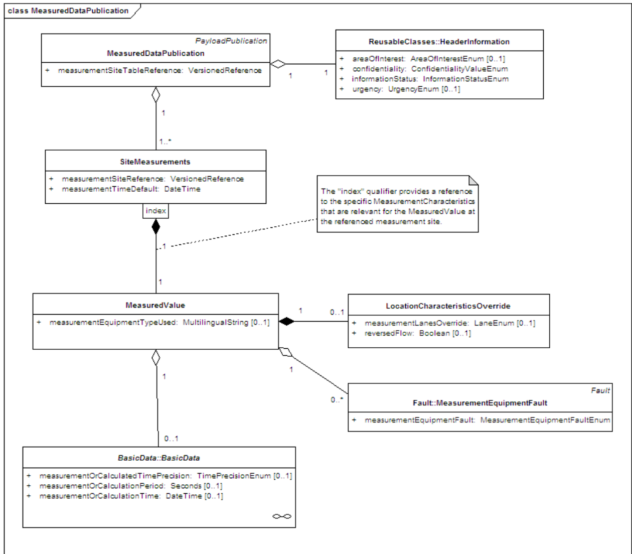
Obrázek 2 – Model tříd balíčku „MeasuredDataPublication”
