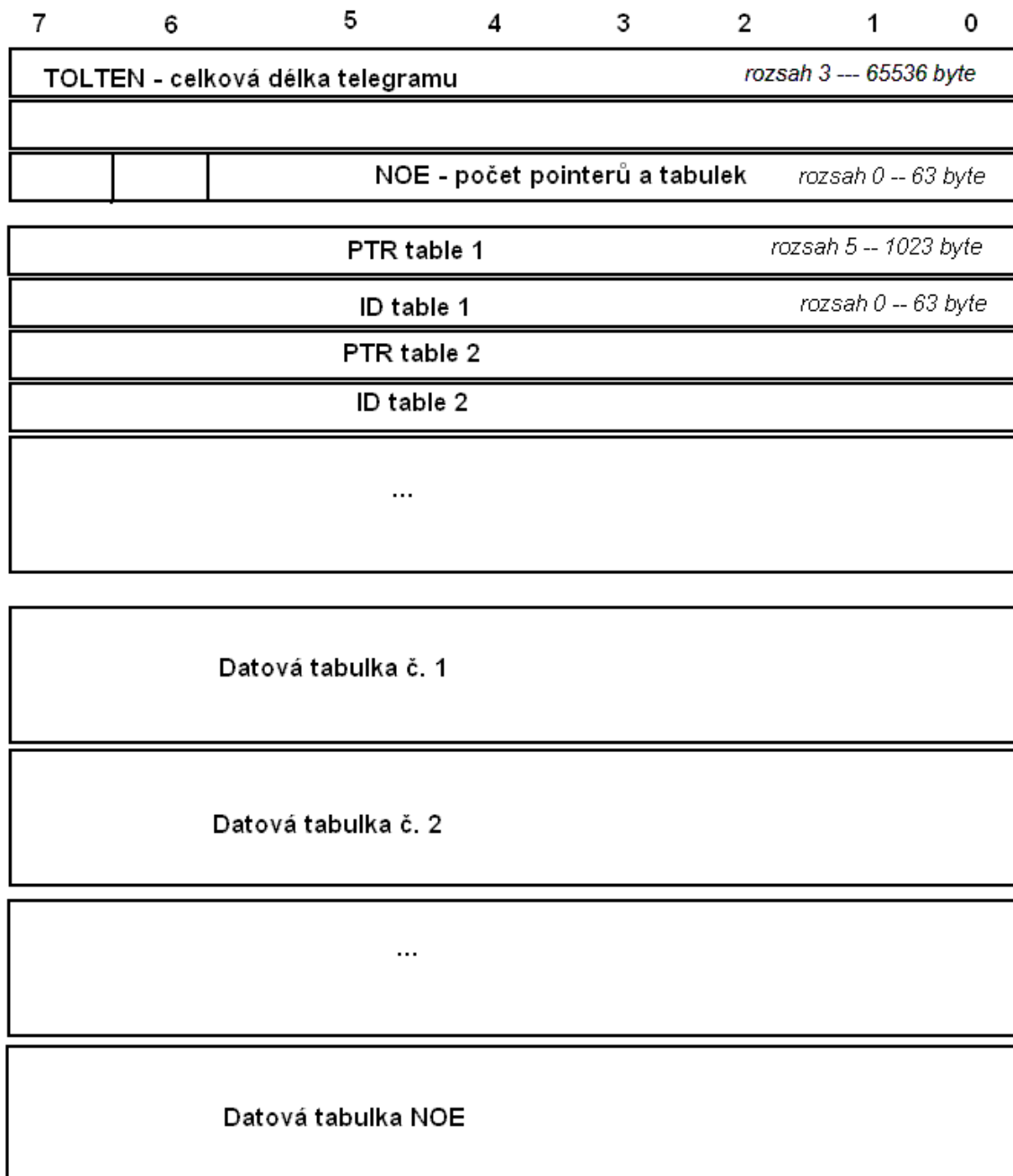
Obrázek 1 – Struktura telegramu
