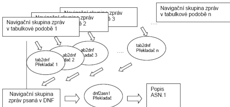
Obrázek 2 – Převod tabulkové podoby skupiny navigačních zpráv do formátu ASN.1
