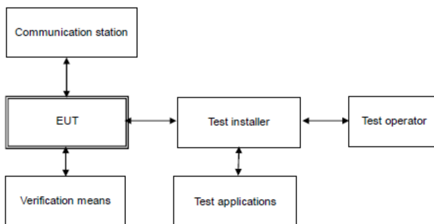
Obrázek 2 – Schéma celého systému pro prokazování shody
