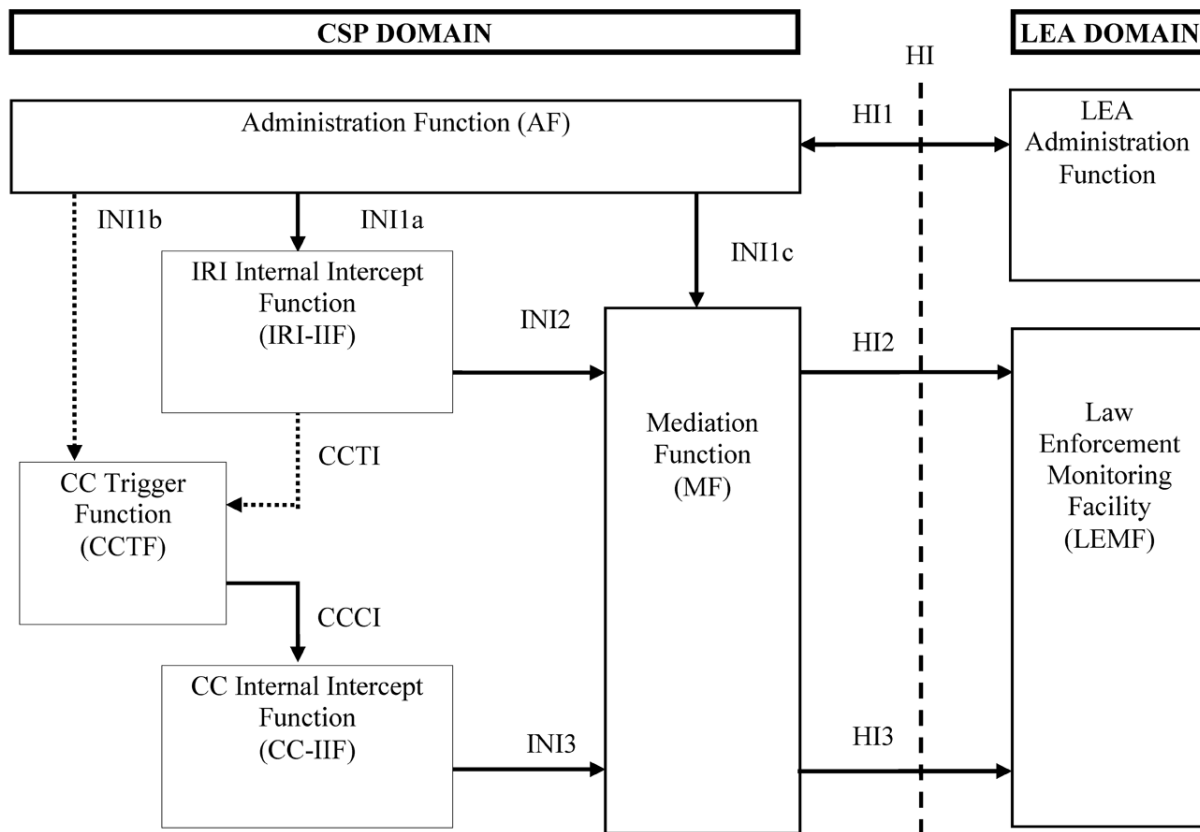
Obrázek 3 – Schéma referenčního modelu, který znázorňuje vztahy mezi provozovatelem komunikační služby a legislativní agenturou dohlížející na procesy
