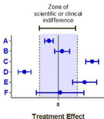
Obrázek 5 – Možné vztahy mezi hodnotami ze 6 různých laboratoří a kalibračními daty oblasti indifferencie
