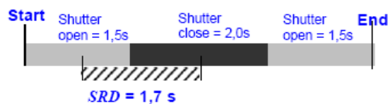
Obrázek A.1 – Načasování vazby zpoždění odezvy systému na intervaly zraku a okluze
